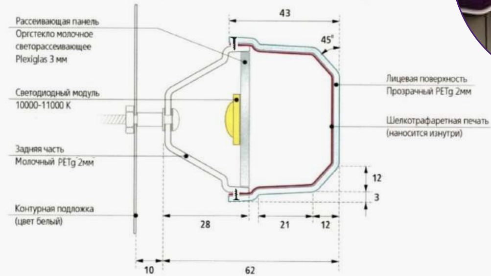
Разрез А-А Стандарт 300
